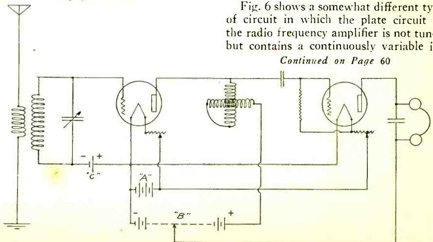
Fig. 6. Regenerative Variometer-Coupled R. F. Amplifier
