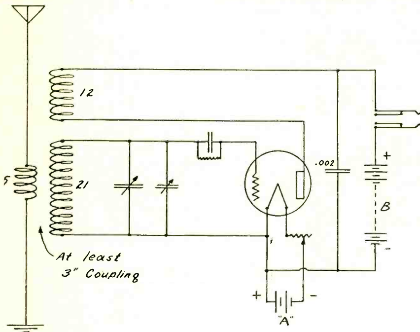
Fig. 1. Wiring Diagram
