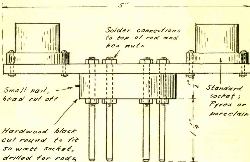
50-Watt Socket Adapter
